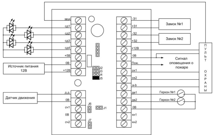
Рис.6. Схема подключения контроллера для режима прохода № 5, 6
