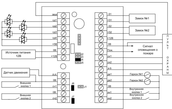
Рис.3. Схема подключения контроллера для режима прохода № 1
