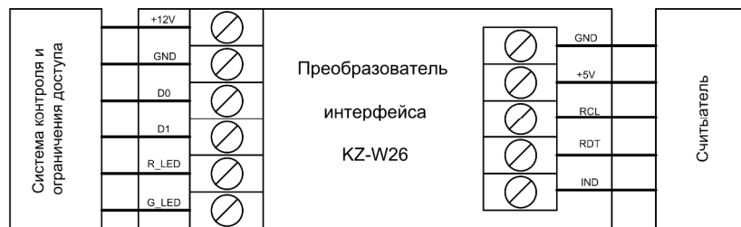
Рисунок 1. Схема подключения преобразователя интерфейсов
