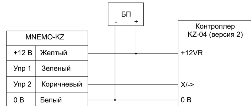
Рис.4 Схема подключения к контроллеру KZ-04
