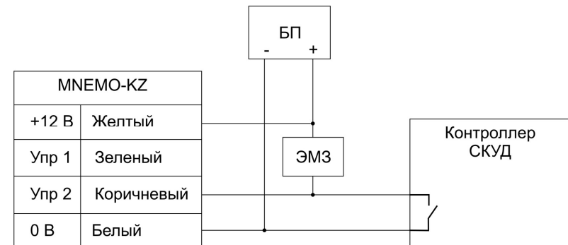
Рис.3 Схема подключения к нормально закрытому замку
