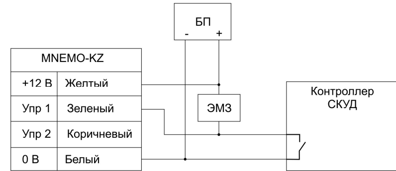
Рис.2 Схема подключения к нормально открытому замку
